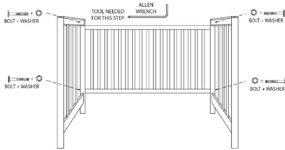
CRIB - STEP 1
