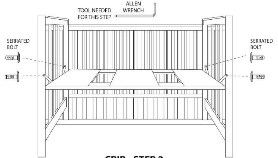
CRIB - STEP 2
