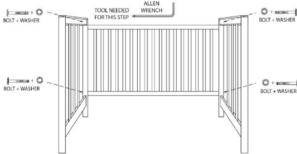
CRIB - STEP 1
